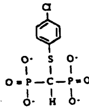
Tiludronate
